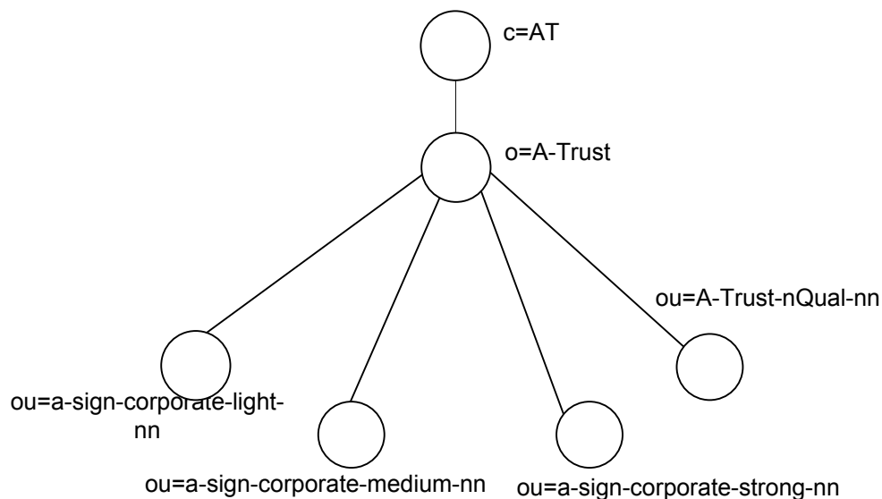
Abbildung 2 a.trust Verzeichnisbaum
